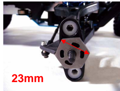
23mm Heavy-duty 23mm Aluminium Radmitnehmer
