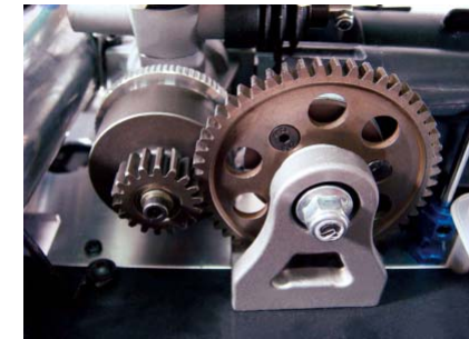
Neue Kupplungsglocke, gehärtetes Stahlhauptzahnrag und Stahl Getrieberäder
